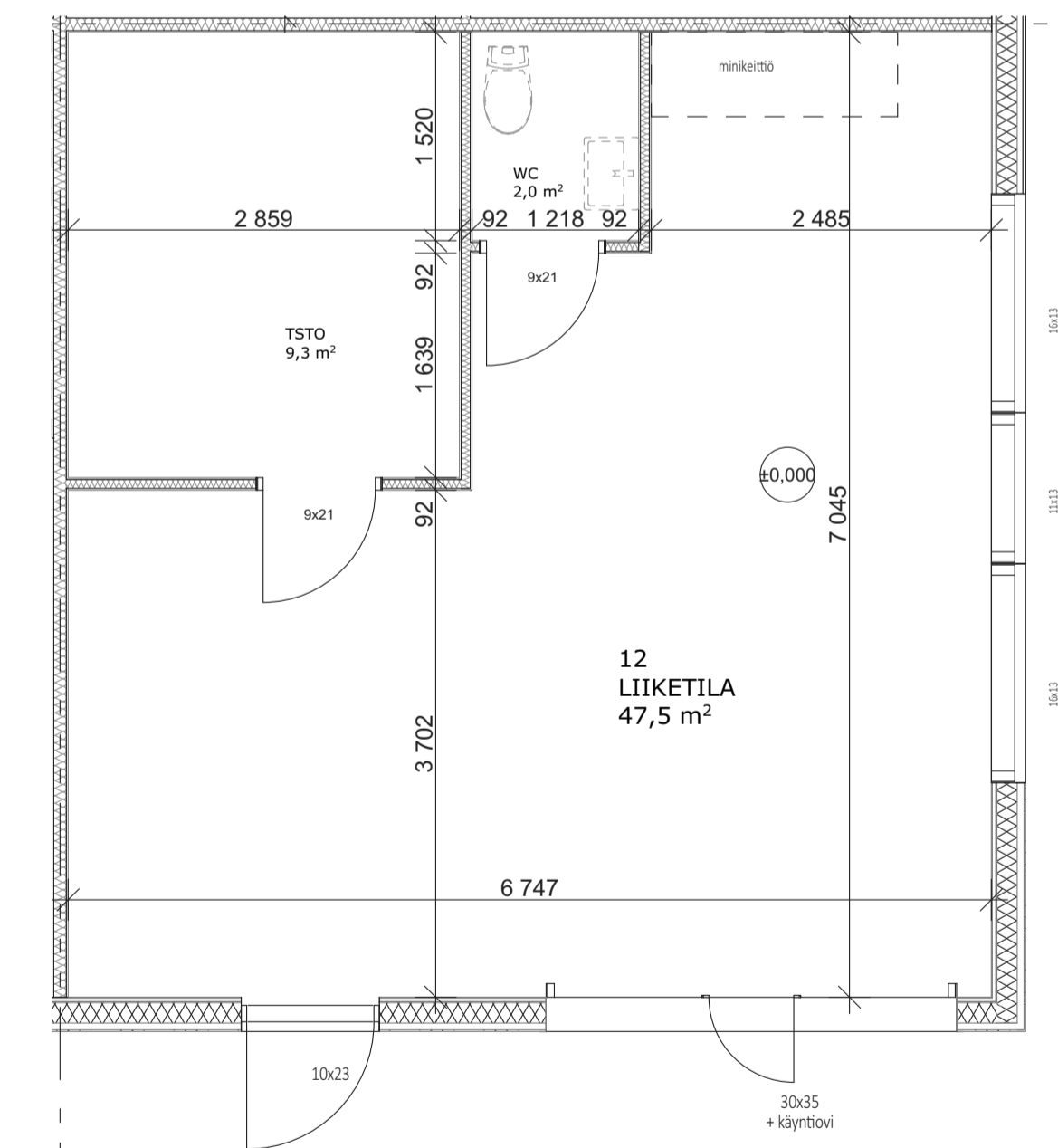
LIIKETILA 12 47,5 m 2
