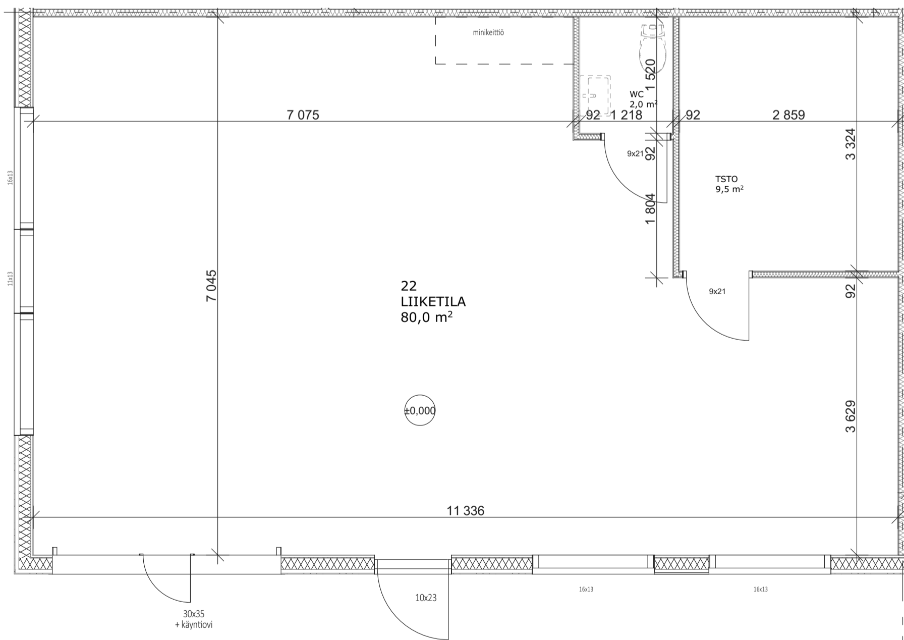
LIIKETILA 22 80,0 m 2
