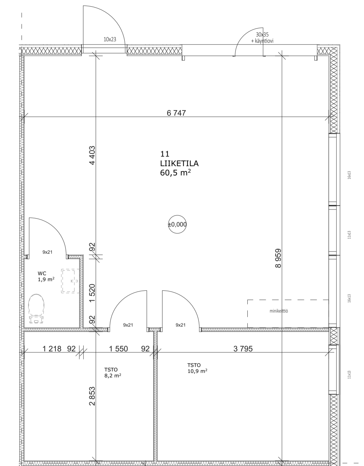
LIIKETILA 11 60,5 m 2
