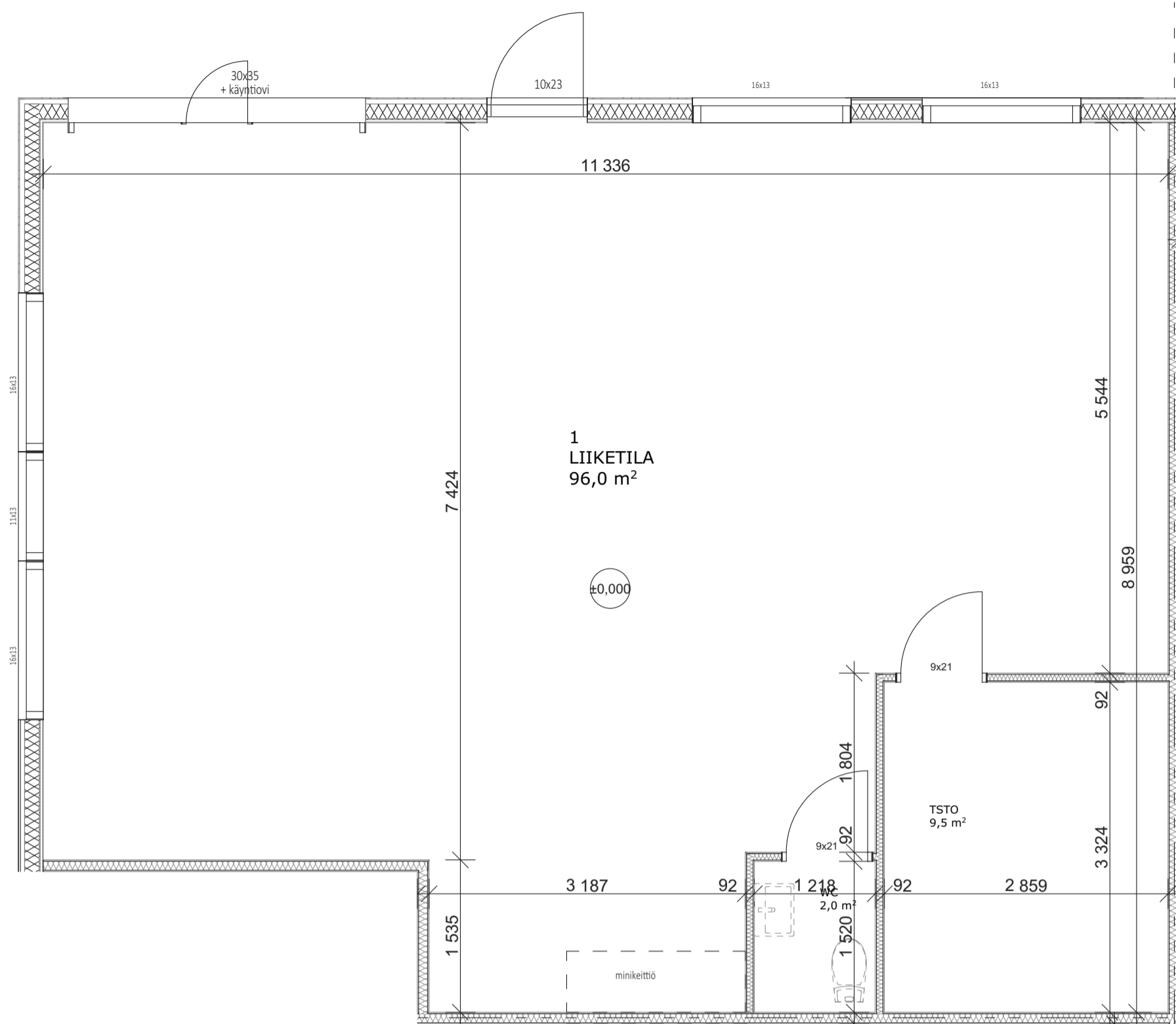
LIIKETILA 1 96,0 m 2
